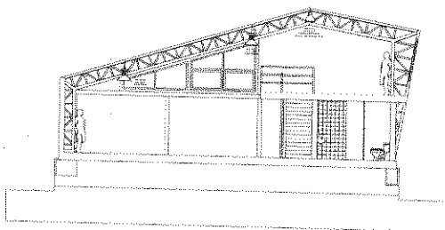
CORTE SALÓN MULTIDEPORTIVO ESCALA 1:50
